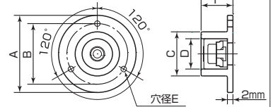
R25T φ42×H11.5
